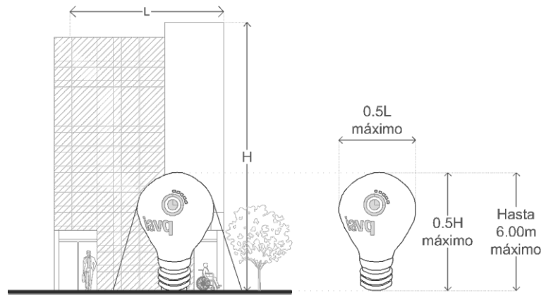
Dimensiones Máximas de Anuncios Inflables.
