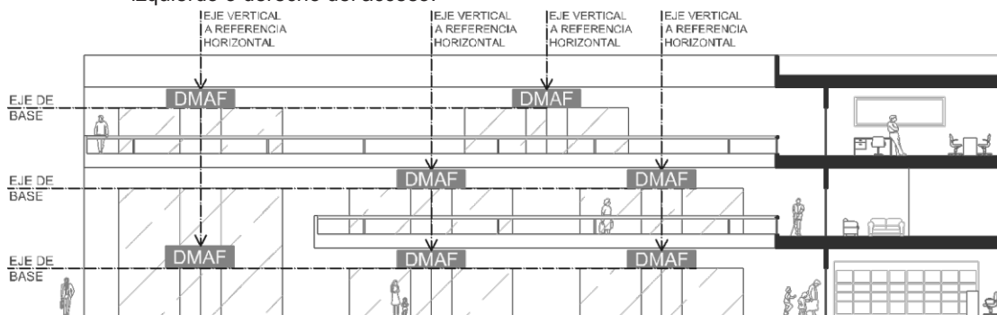
Ilustración que muestra los ejes verticales y horizontales de colocación. Para este caso, el eje vertical se referencia al centro de las puertas de accesos
