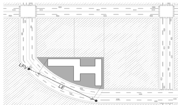
Lado a Vía Pública (LV) y Línea de Frente a Vía Pública (LFV)
