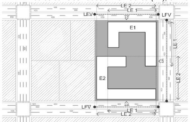
Largos de Edificación (LE) medidos sobre Líneas de Frente a Vía Pública (LFV)
