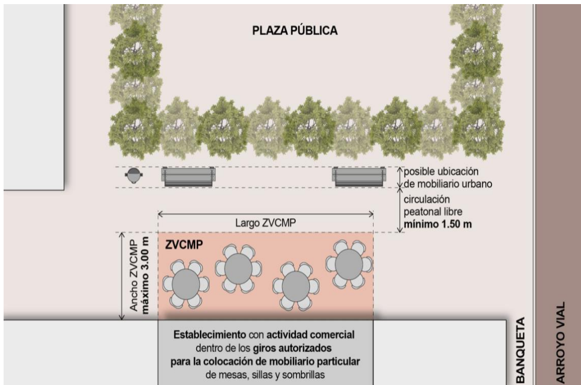
Zona Viable para Colocación de Mobiliario Particular (ZVCMP) en plazas públicas
