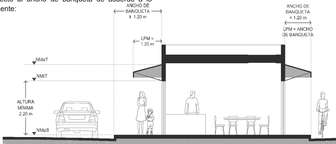
Esquema que ilustra las medidas máximas y mínimas que norman los toldos
