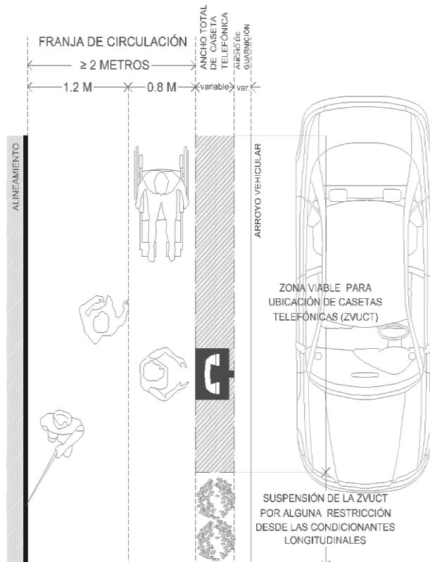
Esquema Banquetas Amplias en planta
