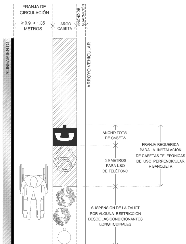
Esquema Banquetas Mínimas en planta
