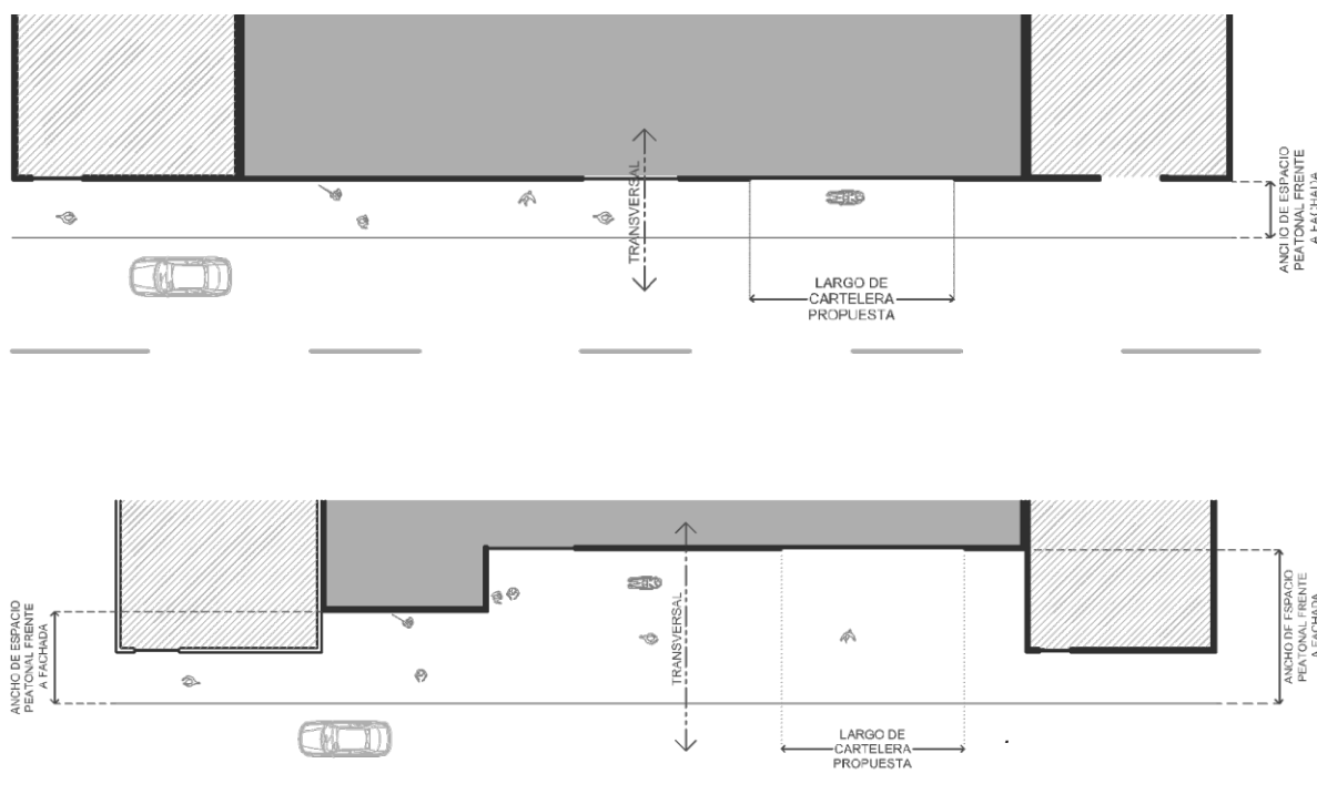
Plantas que muestran los anchos del espacio peatonal frente al inmueble sede de espectáculos públicos
