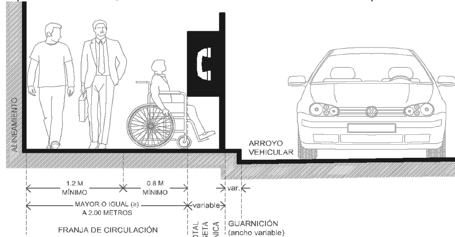
Esquema Banquetas Amplias en alzado
