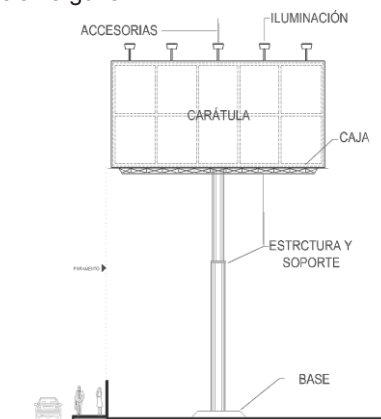
Elementos Integrantes de los anuncios autosoportados.
