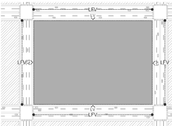
Lados a Vía Pública (LV) y Líneas de Frente a Vía Pública (LFV)
