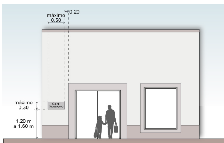
Esquema de Dimensiones Máximas de Anuncio Denominativo en Fachada:
