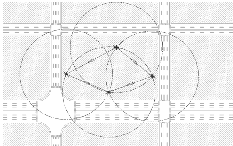
Formato de medición del DMA dentro de un mismo predio.
