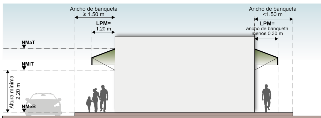
Esquema de medidas máximas y mínimas para la colocación y proyección de toldos
