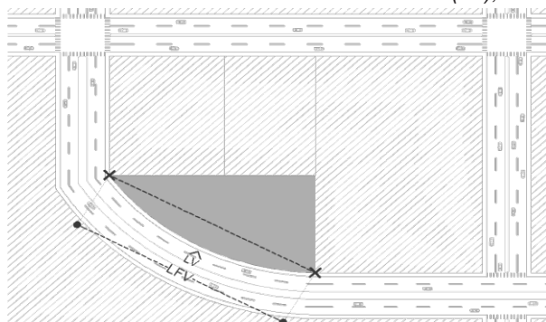
Largo de edificación (LE) medido sobre Línea de Frente a Vía Pública (LFV)
