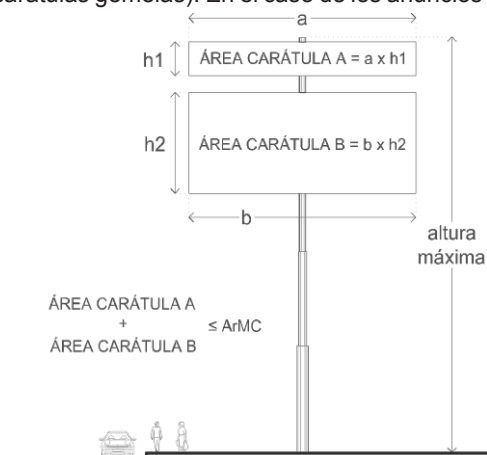
Cálculo del Área de Carátula en anuncios autoportados con dos niveles.
