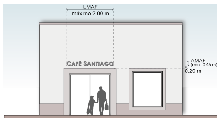
Esquema de Dimensiones Máximas de Anuncio Denominativo en Fachada:
